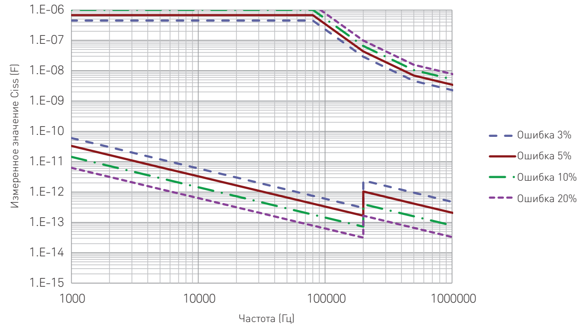
Точность измерения Ciss для устройства с 3 выводами Cgs:Cds:Cgd = 1:0.1:0.01
